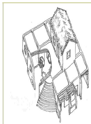
Traditionele compound in leembouw. Tekening van Yere's huis.
